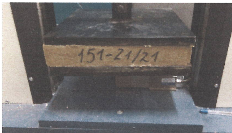
Рисунок 5 – Проведення випробування міцності на стиск при 10% деформації зразків теплоізоляційного матеріалу марки «ТЕХНОРУФ В ОПТИМА»
